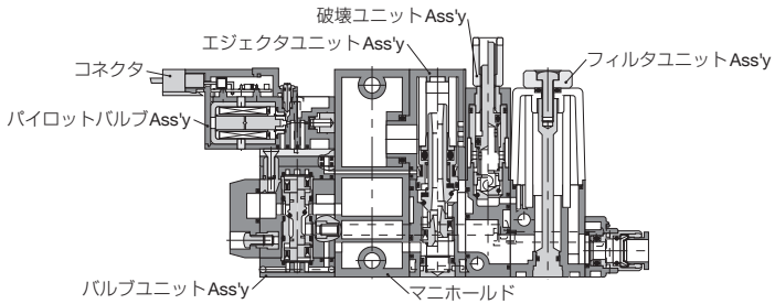
マニホールドタイプ 圧力センサ無し
