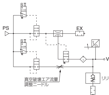
回路図 (VJ□□B ノーマルクローズタイプ)
