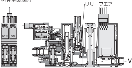
④ 真空破壊時
