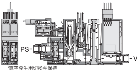
③ 真空保持状態
