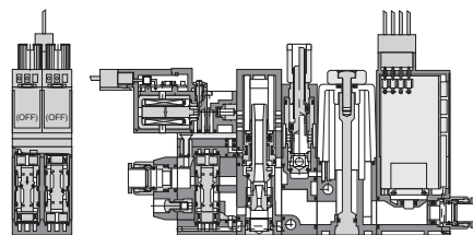
③ 真空保持状態
