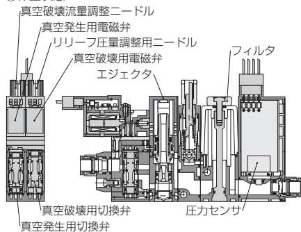
③ 真空保持状態
