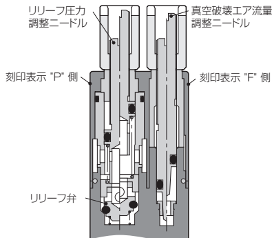
真空破壊ユニット部構造図
