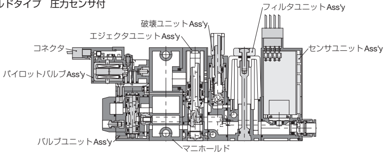
マニホールドタイプ 圧力センサ付
