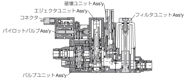
単体タイプ 圧力センサ無し
